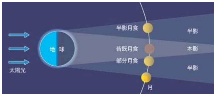
▲月食のしくみ（国立天文台ホームページを参考に作成）
